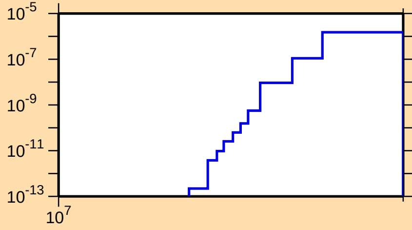
\sigma vs. E for ^{73}\text{Kr}(\text{mt } 34)
