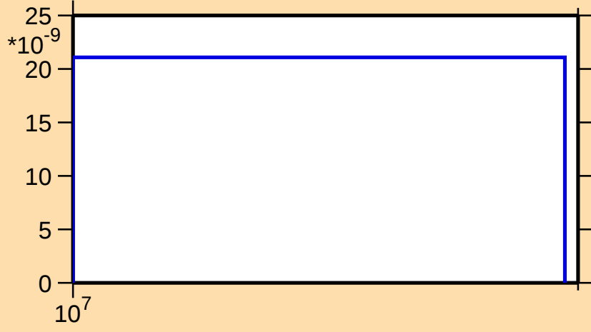
\sigma vs. E for ^{73}\text{Kr}(\text{mt } 34)
