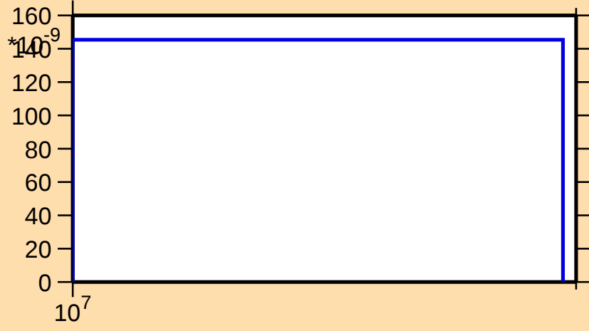
\sigma vs. E for ^{73}\text{Kr}(\text{mt } 45)
