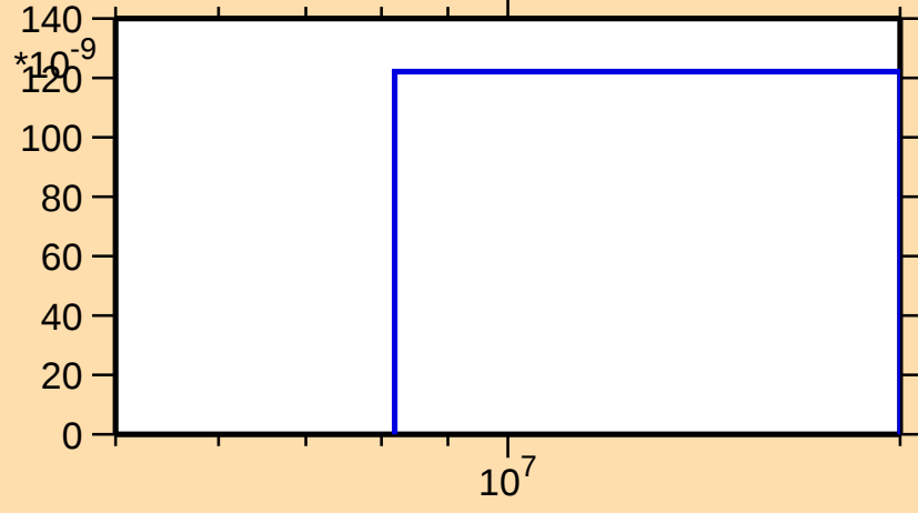
\sigma vs. E for ^{73}\text{Kr}(\text{mt } 45)
