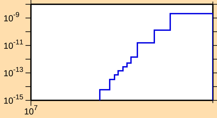
\sigma vs. E for ^{161}\text{Ta}(\text{mt } 34)
