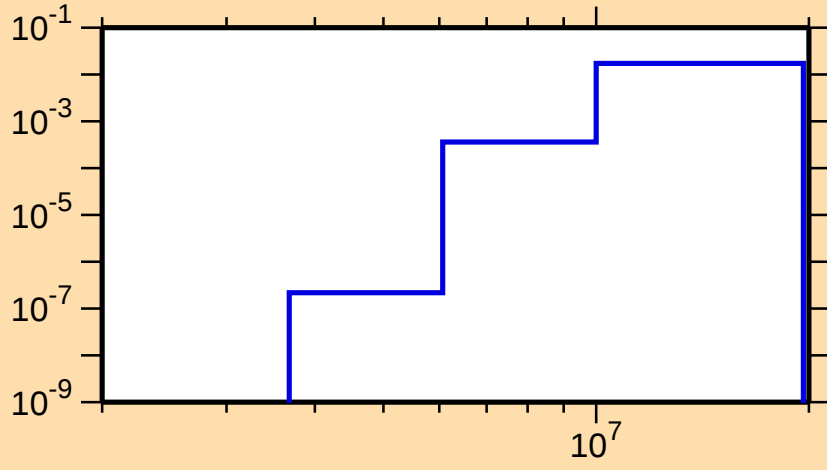
\sigma vs. E for ^{161}\text{Ta}(\text{mt } 45)
