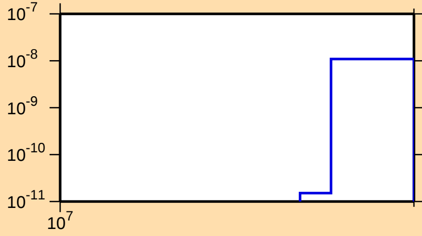
\sigma vs. E for ^{73}\text{As} (mt 45)
