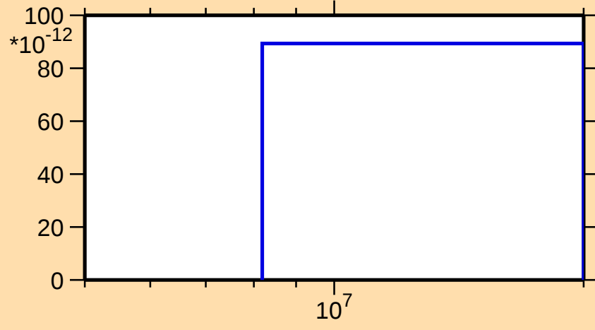
\sigma vs. E for ^{73}\text{As}(\text{mt } 45)
