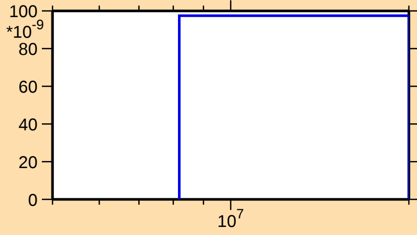
\sigma vs. E for ^{194}\text{Bi}(\text{mt } 45)
