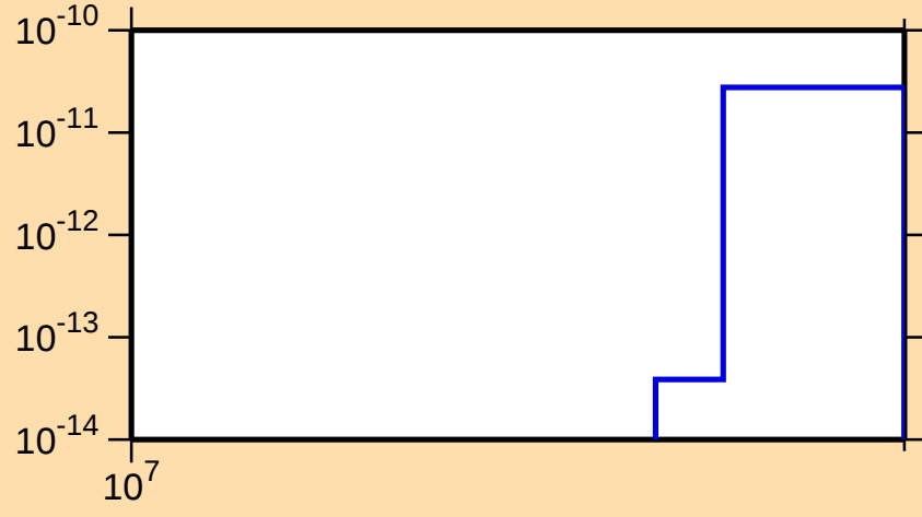
\sigma vs. E for ^{126}\text{Cs} (mt 34)
