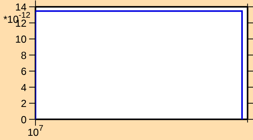
\sigma vs. E for ^{126}\text{Cs} (mt 45)
