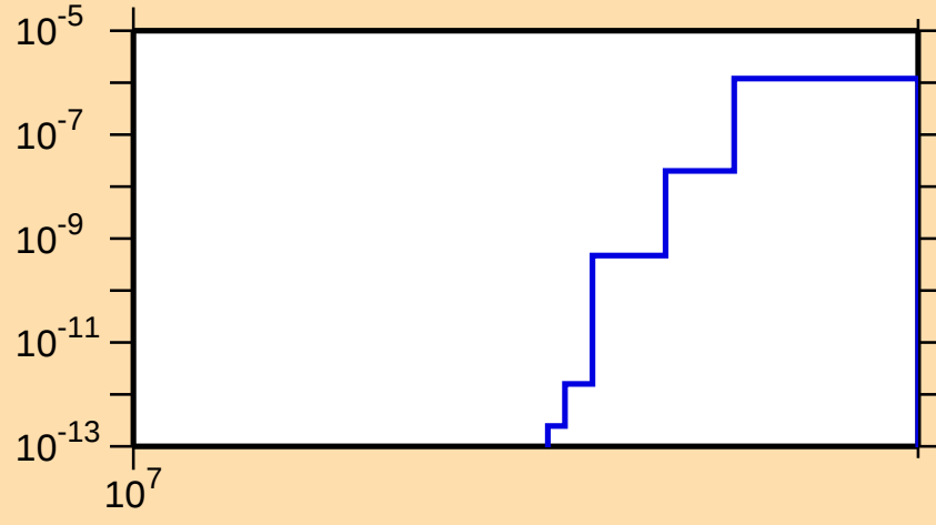
\sigma vs. E for ^{64}\text{Ga}(\text{mt } 34)
