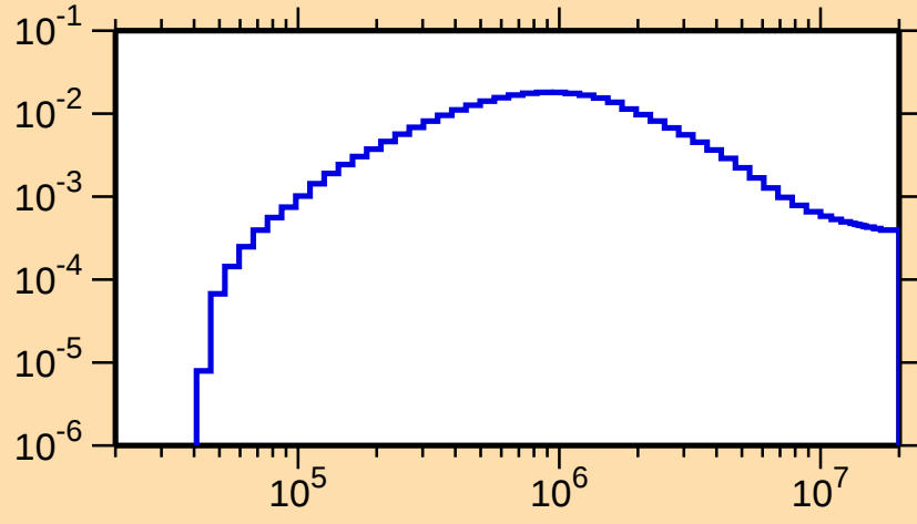
\sigma vs. E for ^{64}\text{Ga}(n,n_1)
