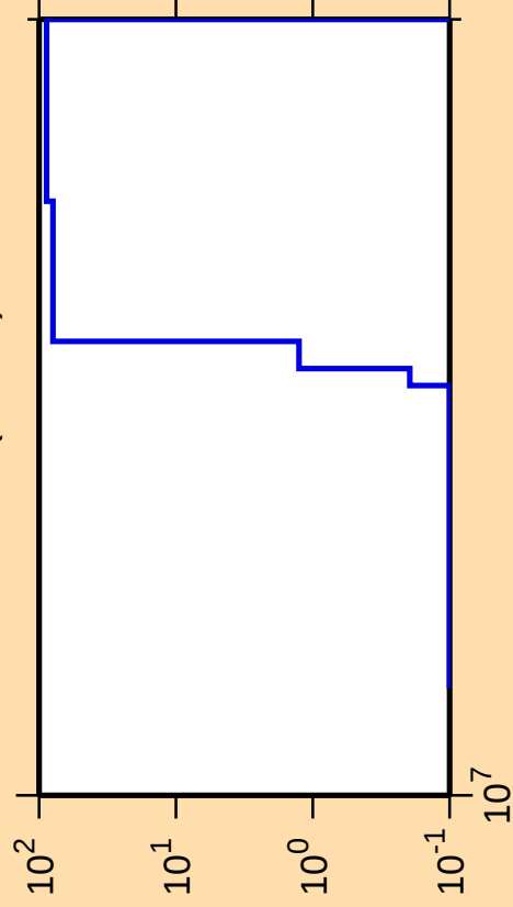
\Delta\sigma/\sigma vs. E for ^{64}\text{Ga}(\text{mt } 34)
