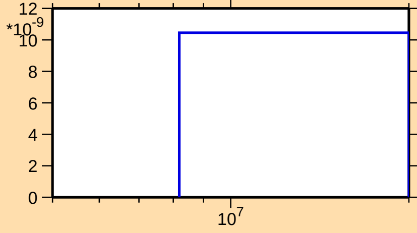
\sigma vs. E for ^{137}\text{Gd}(\text{mt } 34)
