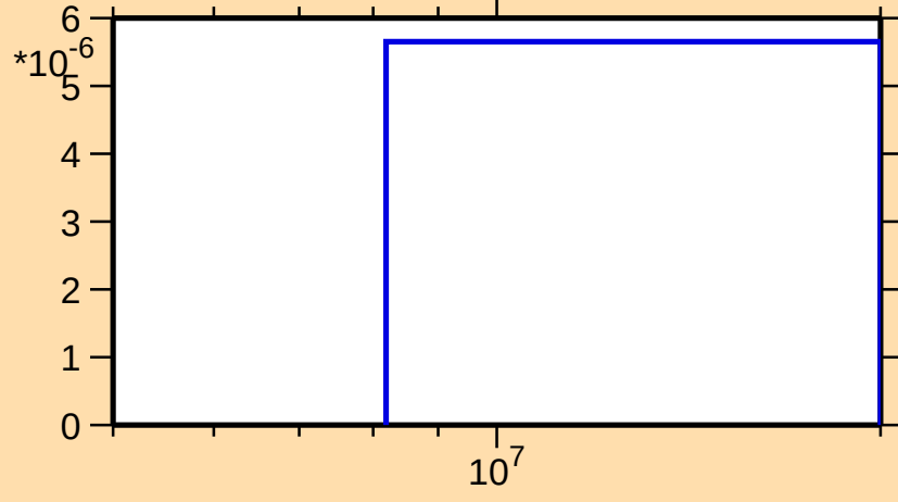
\sigma vs. E for ^{137}\text{Gd}(\text{mt } 45)
