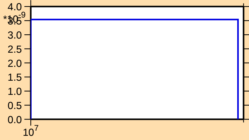
\sigma vs. E for ^{143}\text{Gd}(\text{mt } 45)
