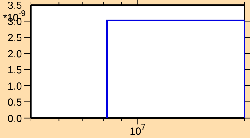
\sigma vs. E for ^{143}\text{Gd}(\text{mt } 45)
