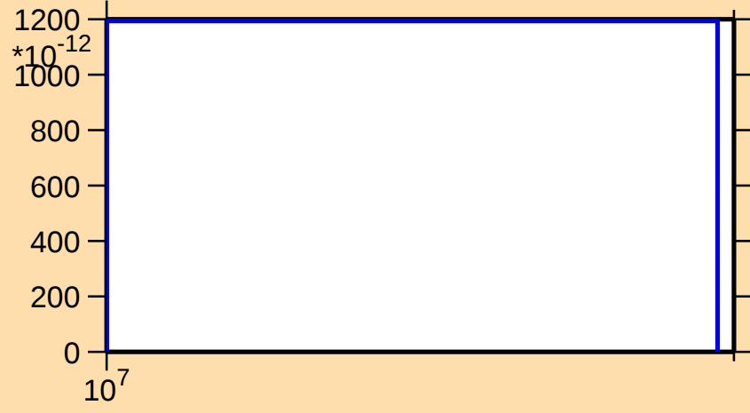
\sigma vs. E for ^{144}\text{Gd}(\text{mt } 45)
