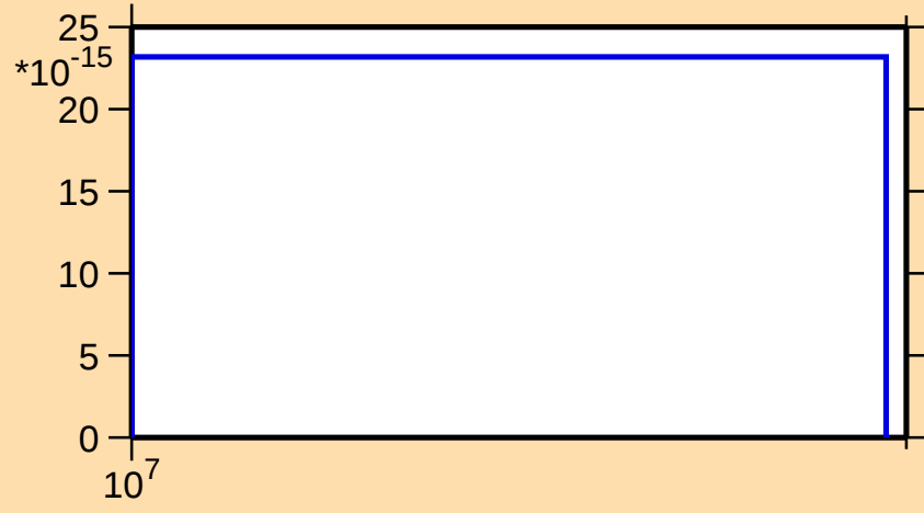
\sigma vs. E for ^{144}\text{Gd}(\text{mt } 34)
