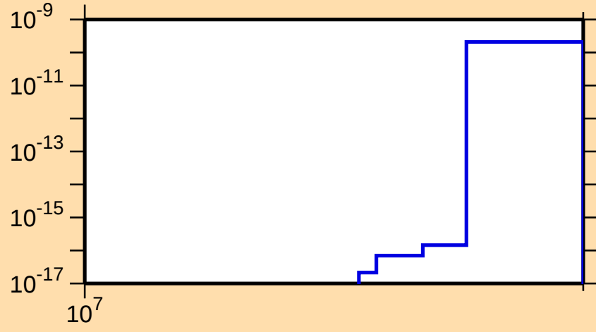
\sigma vs. E for ^{66}\text{Ge}(\text{mt } 34)
