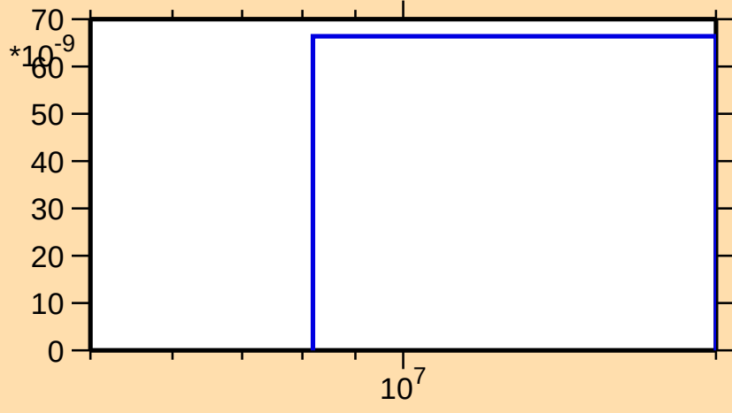
\sigma vs. E for ^{66}\text{Ge}(\text{mt } 45)
