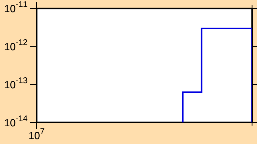
\sigma vs. E for ^{254}\text{Md}(\text{mt } 34)
