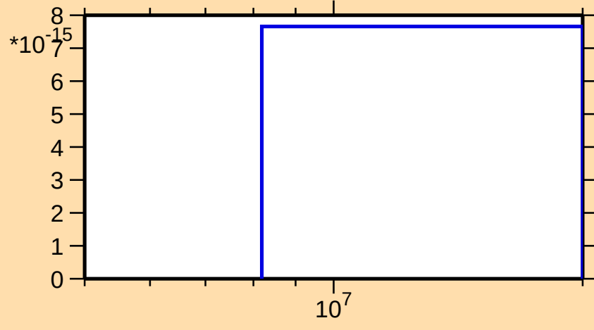
\sigma vs. E for ^{257}\text{Md}(\text{mt } 42)
