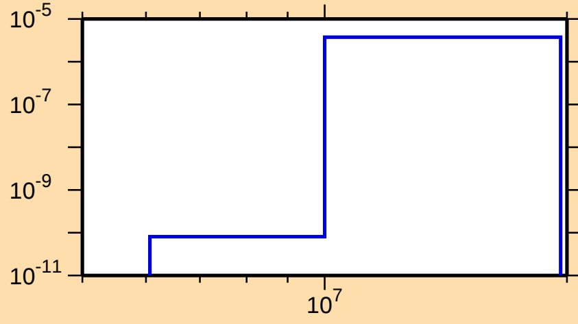
\sigma vs. E for ^{196}\text{Po}(\text{mt } 45)
