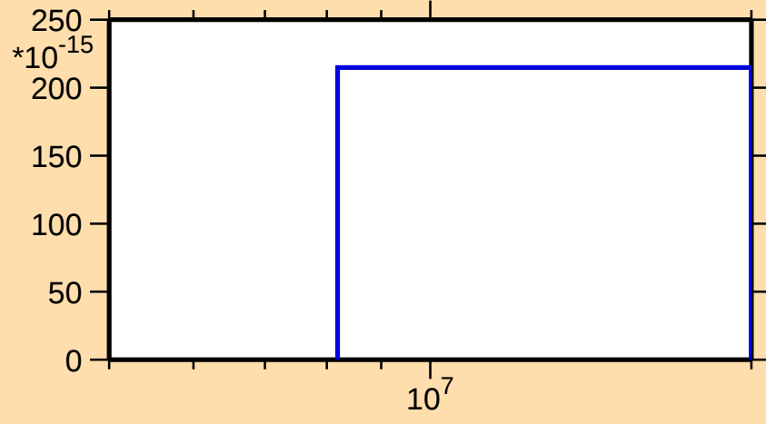
\sigma vs. E for ^{196}\text{Po}(\text{mt } 34)
