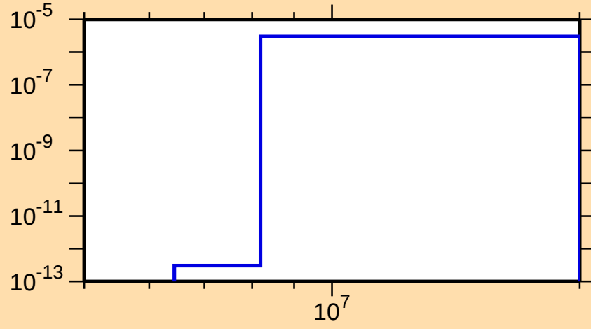
\sigma vs. E for ^{196}\text{Po}(\text{mt } 45)
