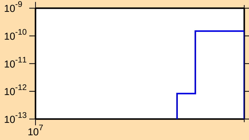
\sigma vs. E for ^{208}\text{Po}(\text{mt } 45)
