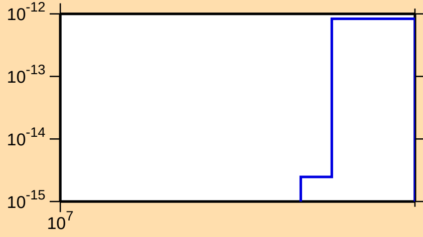
\sigma vs. E for ^{208}\text{Po}(\text{mt } 34)
