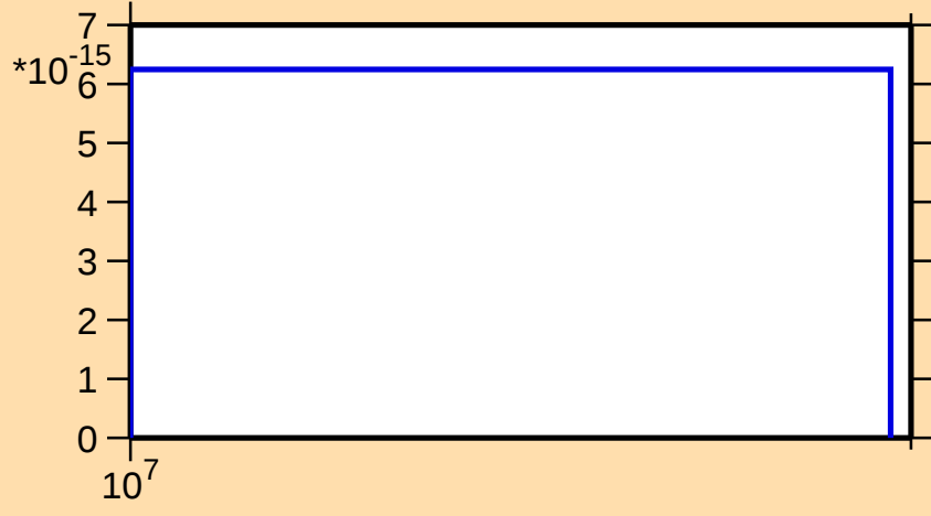
\sigma vs. E for ^{208}\text{Po}(\text{mt } 34)
