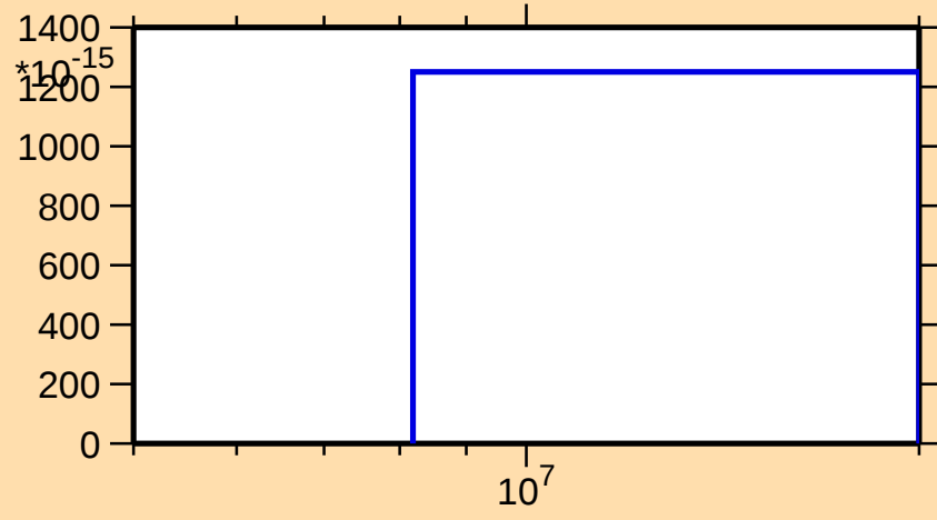
\sigma vs. E for ^{208}\text{Po}(\text{mt } 45)
