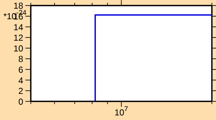
\sigma vs. E for ^{208}\text{Po}(\text{mt } 42)
