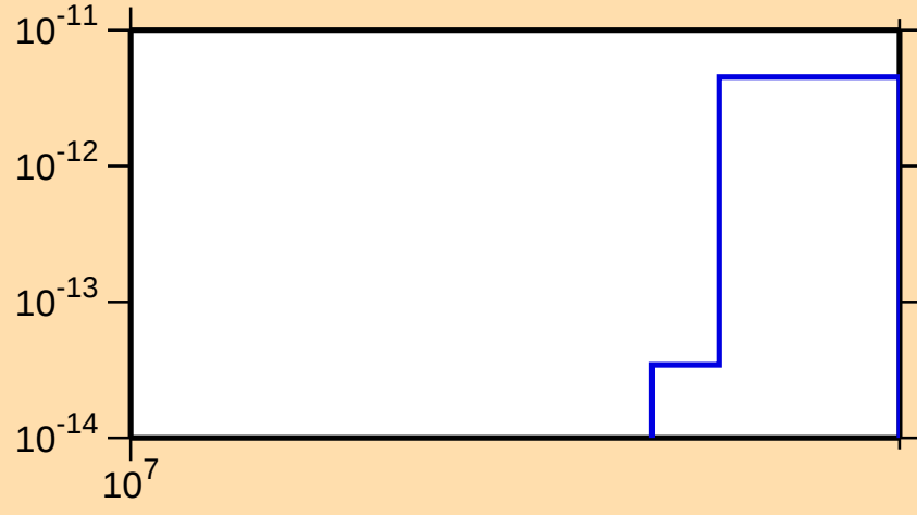
\sigma vs. E for ^{189}\text{Pt}(\text{mt } 34)
