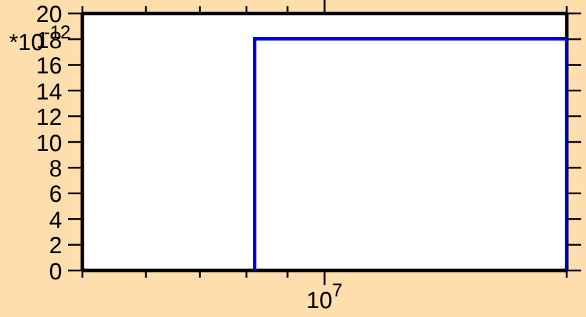
\sigma vs. E for ^{167}\text{Re}(\text{mt } 34)
