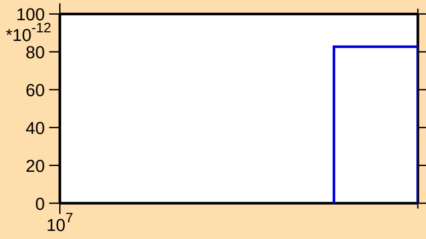
\sigma vs. E for ^{33}\text{S} (mt 34)
