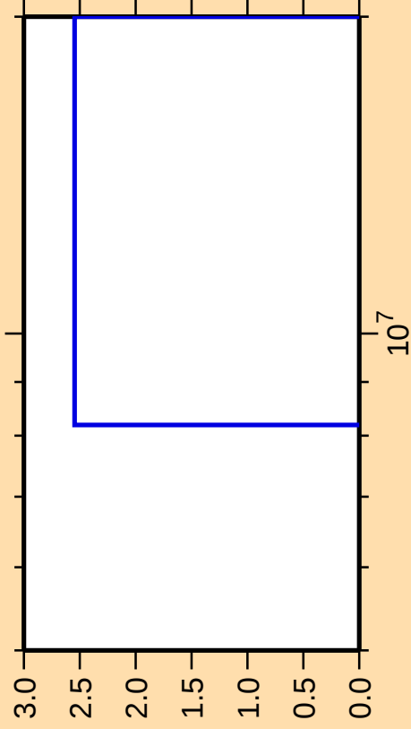
\Delta\sigma/\sigma vs. E for ^{33}\text{S}(\text{mt } 34)
