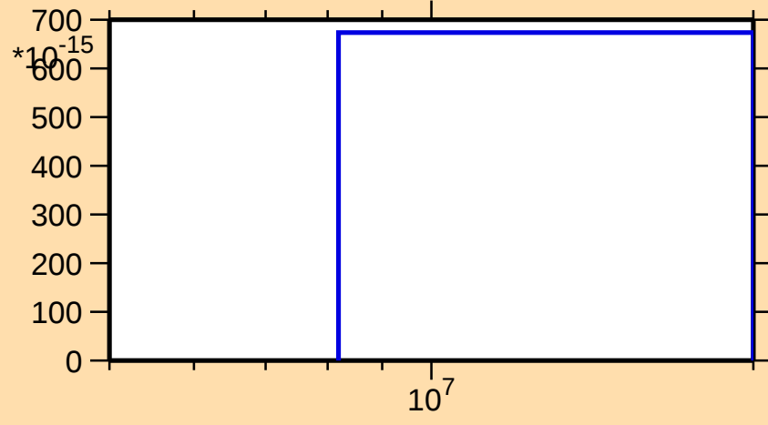
\sigma vs. E for ^{33}\text{S}(\text{mt } 34)
