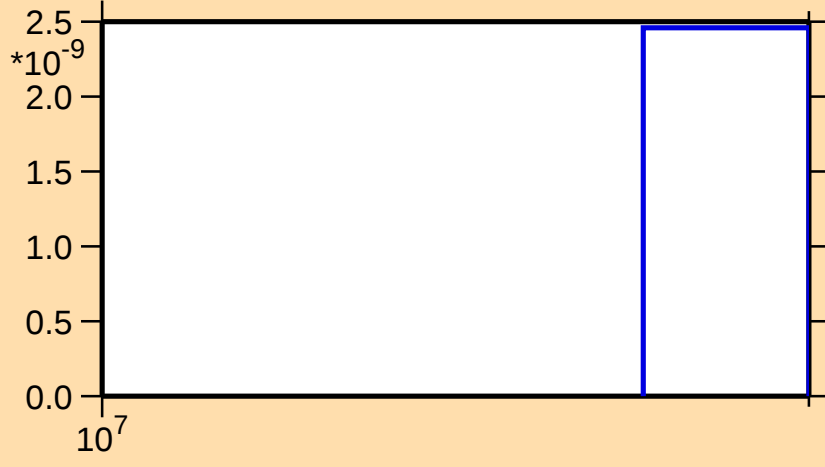
\sigma vs. E for ^{26}\text{Si}(\text{mt } 34)
