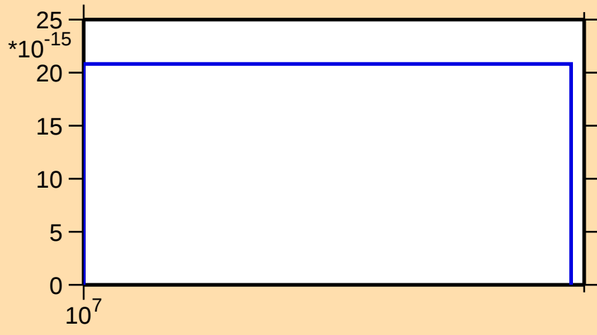
\sigma vs. E for ^{147}\text{Sm}(\text{mt } 34)
