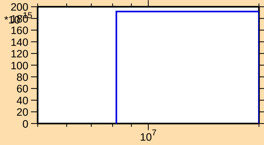
\sigma vs. E for ^{147}\text{Sm}(\text{mt } 45)
