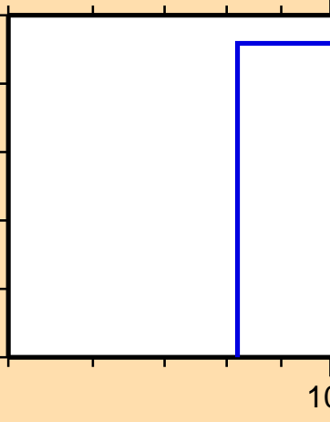
\sigma vs. E for ^{103}\text{Sn}(\text{mt } 34)
