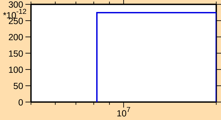
\sigma vs. E for ^{167}\text{W}(\text{mt } 34)
