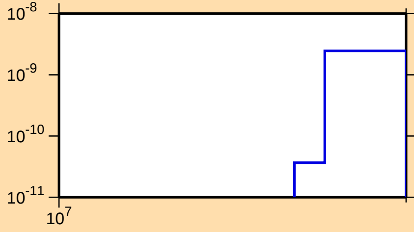
\sigma vs. E for ^{116}\text{Xe}(\text{mt } 34)
