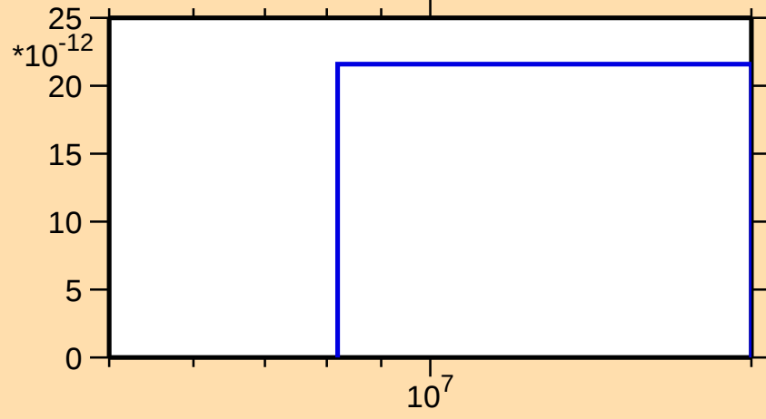
\sigma vs. E for ^{116}\text{Xe}(\text{mt } 34)
