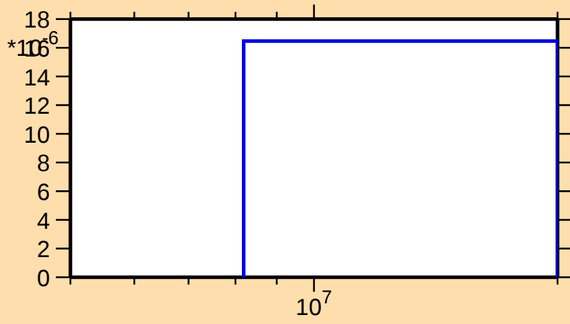
\sigma vs. E for ^{116}\text{Xe}(\text{mt } 45)
