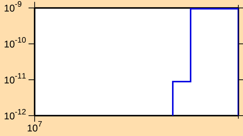
\sigma vs. E for ^{121}\text{Xe}(\text{mt } 34)
