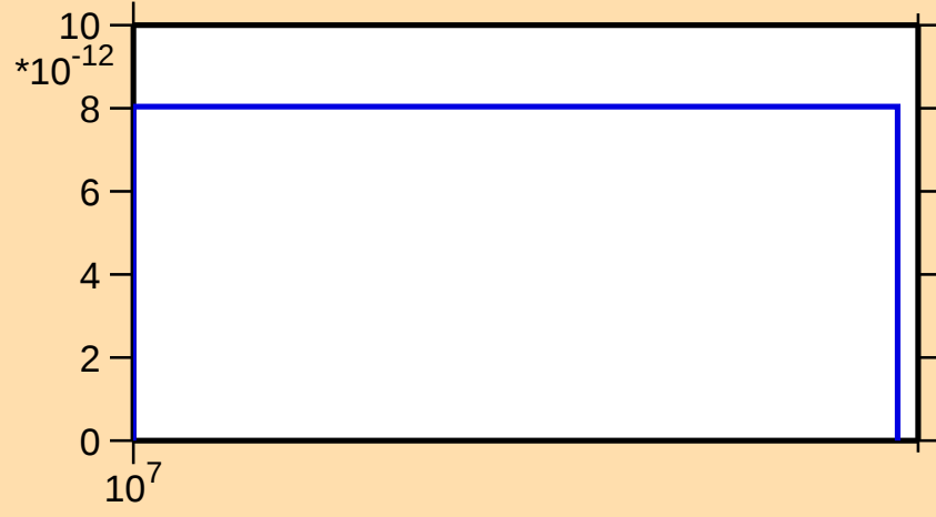
\sigma vs. E for ^{121}\text{Xe}(\text{mt } 34)
