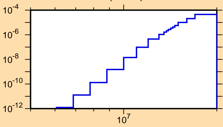
\sigma vs. E for ^{193}\text{Bi}(\text{mt } 45)
