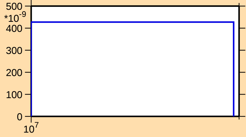
\sigma vs. E for ^{66}\text{Ga}(\text{mt } 45)
