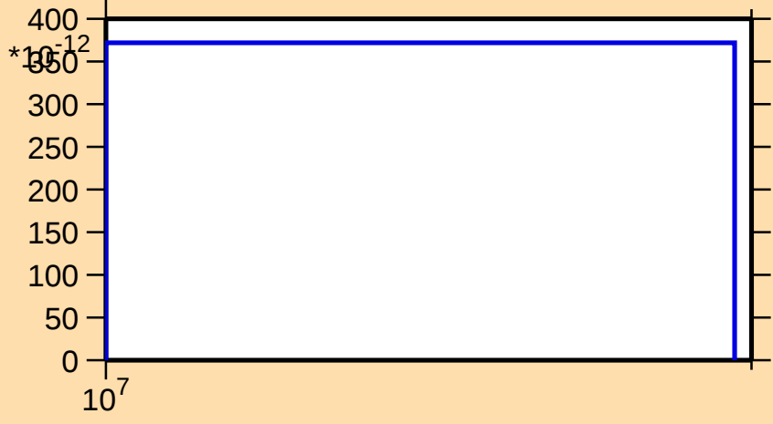
\sigma vs. E for ^{66}\text{Ga}(\text{mt } 34)
