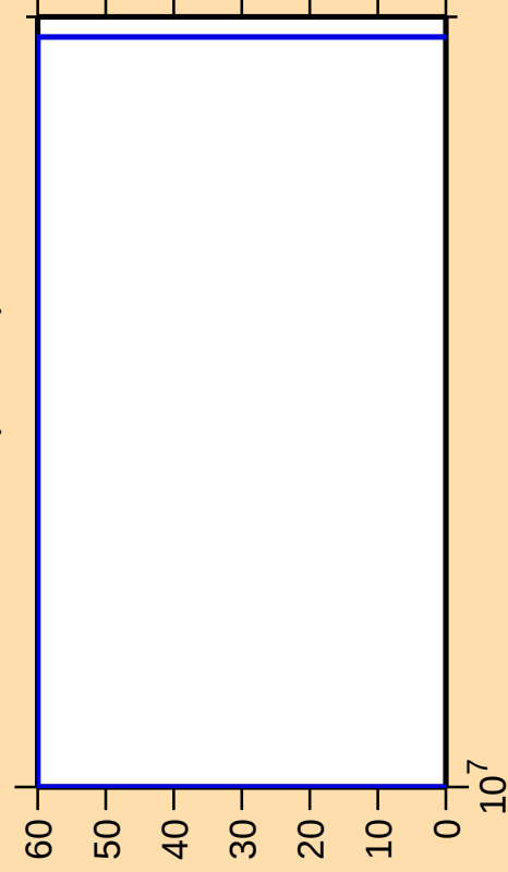
\Delta\sigma/\sigma vs. E for ^{66}\text{Ga}(\text{mt } 45)
