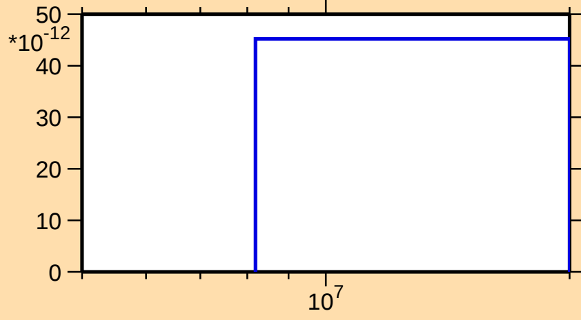
\sigma vs. E for ^{66}\text{Ga}(n,nt)
