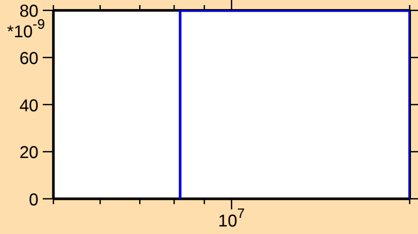
\sigma vs. E for ^{67}\text{Ga}(\text{mt } 45)
