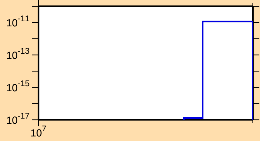
\sigma vs. E for ^{74}\text{Kr}(\text{mt } 34)
