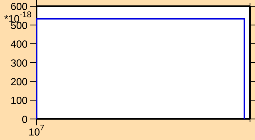
\sigma vs. E for ^{76}\text{Kr}(\text{mt } 34)
