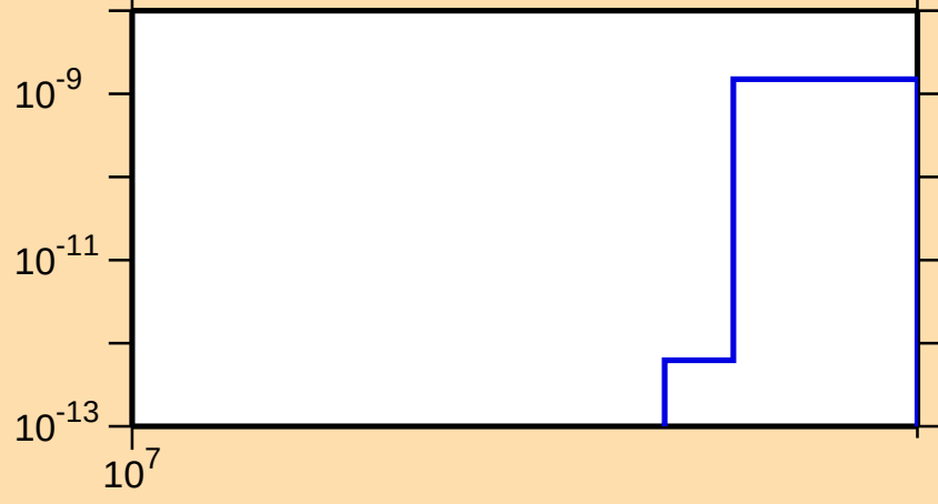
\sigma vs. E for ^{77}\text{Kr}(\text{mt } 34)
