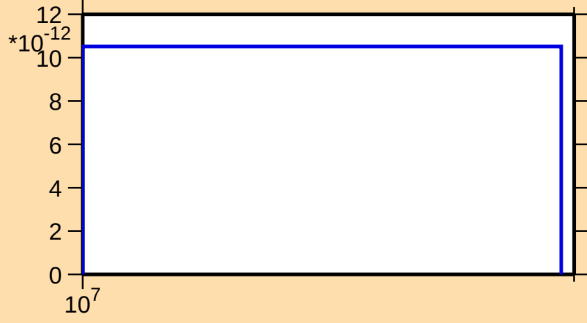
\sigma vs. E for ^{77}\text{Kr}(\text{mt } 34)
