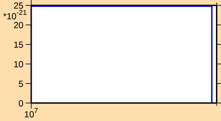
\sigma vs. E for ^{85}\text{Kr}(\text{mt } 34)
