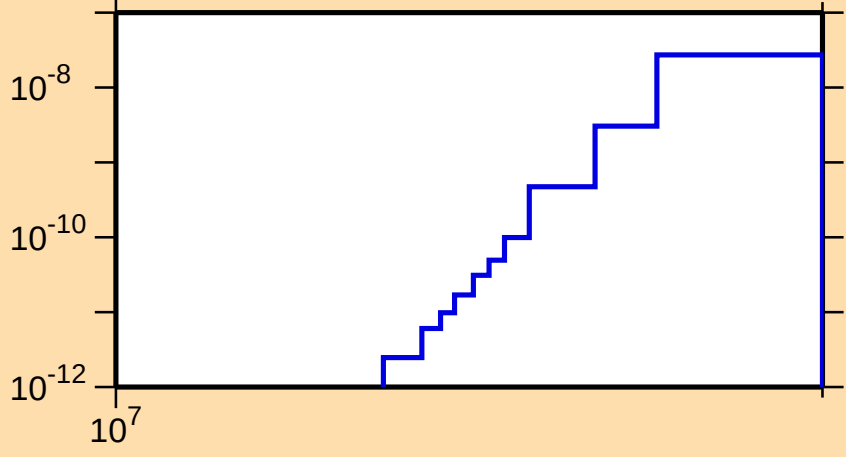
\sigma vs. E for ^{177}\text{Pt}(\text{mt } 34)
