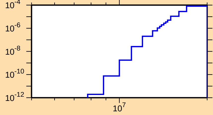
\sigma vs. E for ^{177}\text{Pt}(\text{mt } 45)
