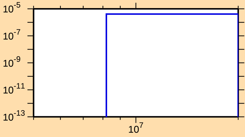
\sigma vs. E for ^{177}\text{Pt}(\text{mt } 45)
