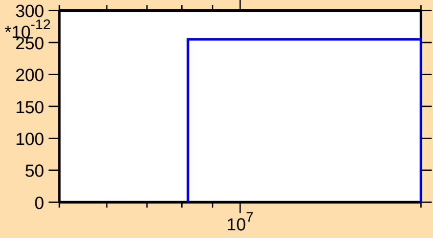
\sigma vs. E for ^{183}\text{Pt}(\text{mt } 45)
