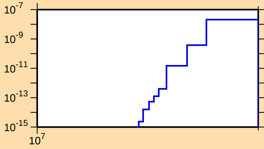
\sigma vs. E for ^{107}\text{Sn}(\text{mt } 34)
