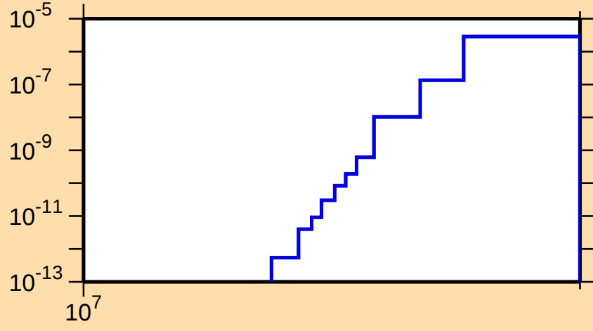
\sigma vs. E for ^{107}\text{Sn}(\text{mt } 45)
